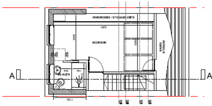
LOFT PLAN
